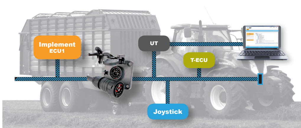
Figura 2: Típico sistema ISOBUS estándar
